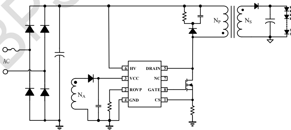
图 1 BP3189B 典型应用电路
