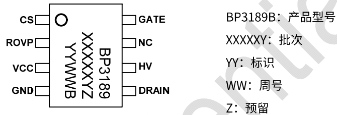
图2 管脚封装图
