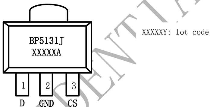
图 2 BP5131JA 管脚封装图
