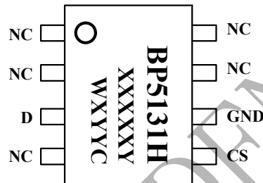
图 2 BP5131HC 管脚封装图
