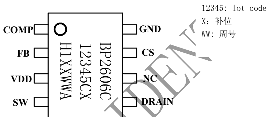
图2 管脚封装图
